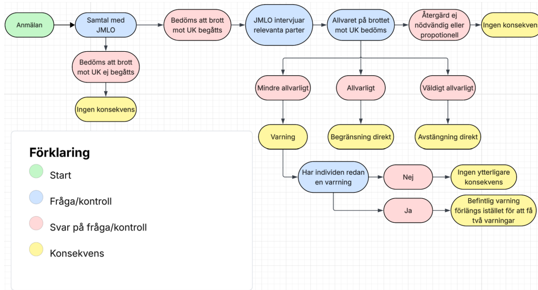
Figur 1: Utredningsprocess. Förklaring: grön = start, blå = fråga/kontroll, rosa = svar på fråga/kontroll, gul = konsekvens.
